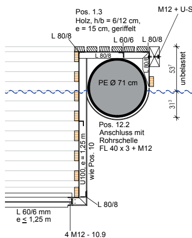
Längsschnitt Schwimmbeckenrand
